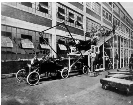
Chaîne de production de la Ford T aux États-Unis
